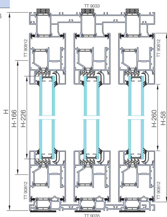
Sez. A-A
