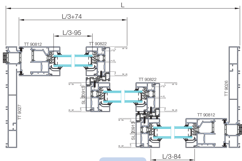
Sez. B-B
