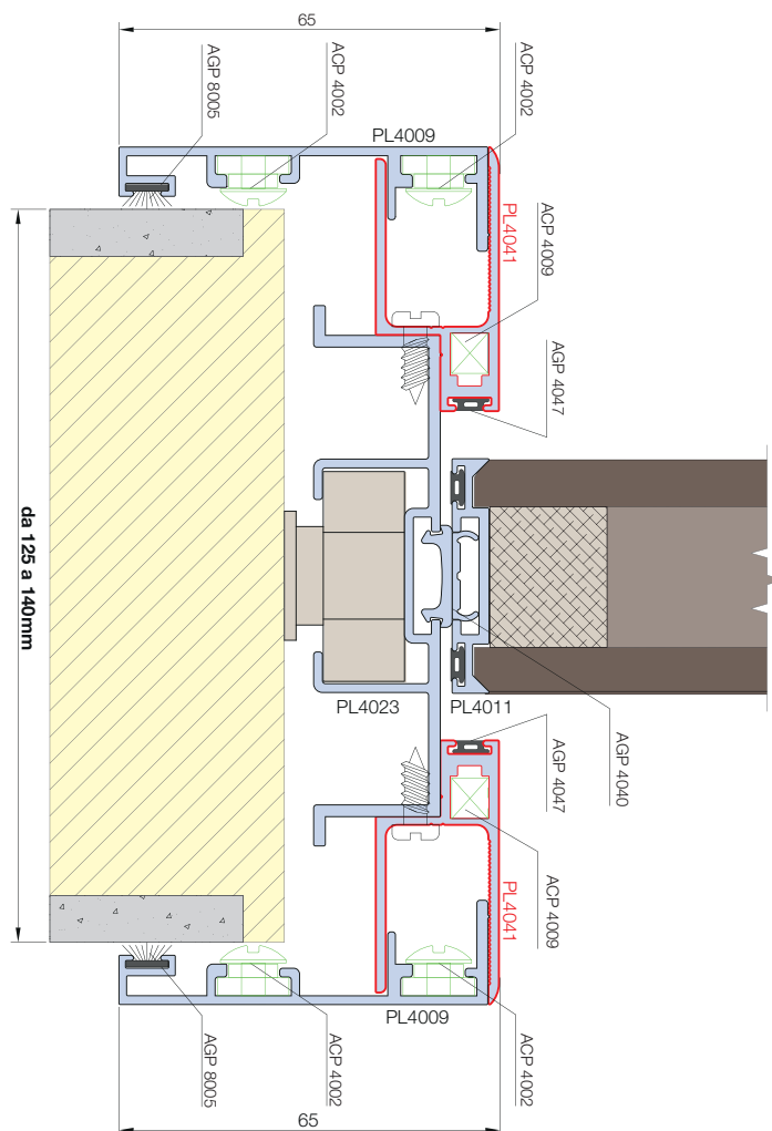
NODO CON TELAIO MAGGIORATO PL 4041
